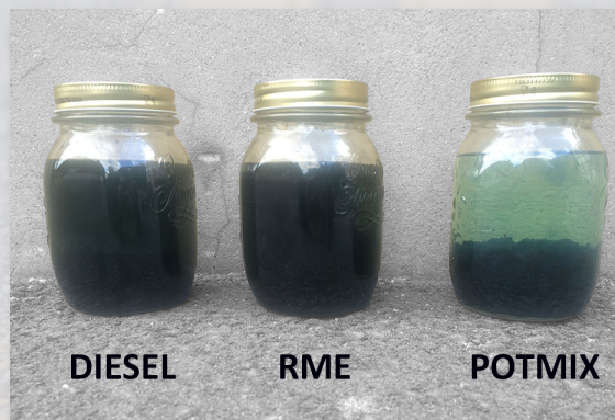
TEST 2: Upplösning av varmasfalt efter fyra timmar
