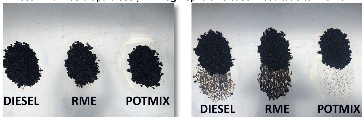
Test 1: Varmasfalt på diesel, RME og Asphalt Release. Resultat efter 2 timer.
